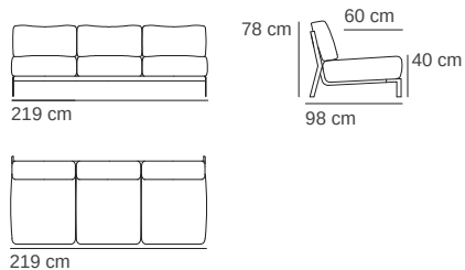
219W × 98D × 78H cm mt 15.1 | 1.98 m³ | 62 kg Module Cod. 033
