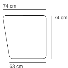
74 / 63W x 74D cm mt 2.1 | 0.33 m³ | 13 kg Seat Cod. SED2
