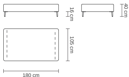
180W × 105D cm Module Cod. DENA180
